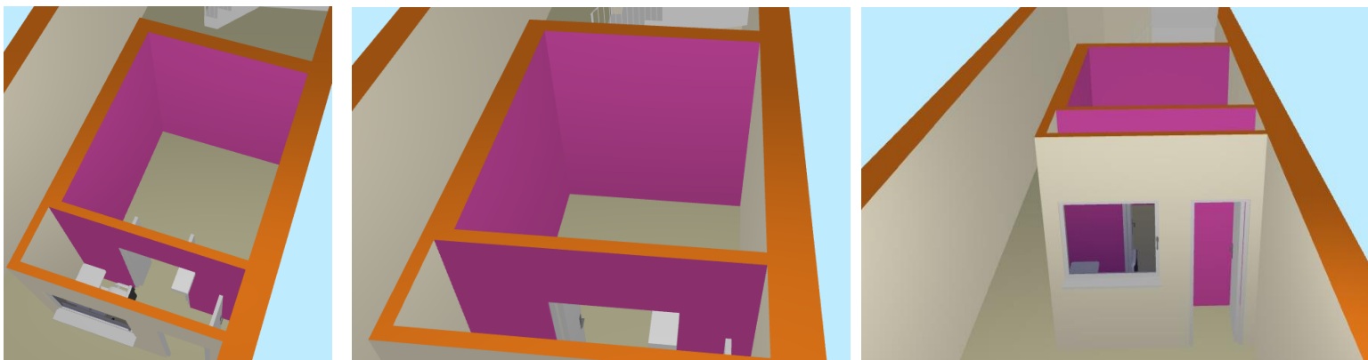
RENCANA DENAH PELETAKAN DINDING TIMBAL 3D
