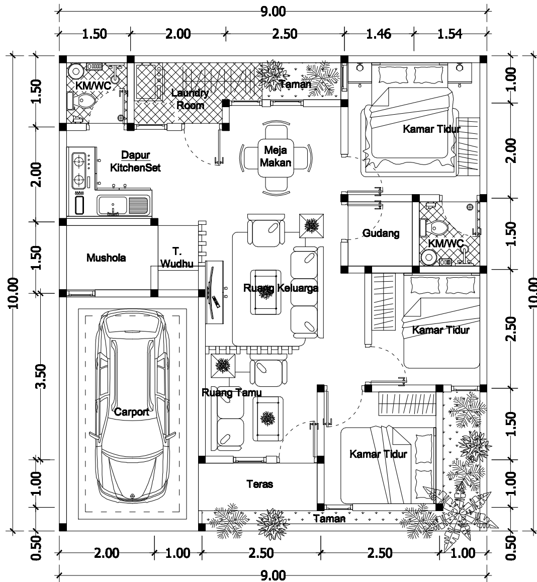
DENAH RUMAH TINGGAL
