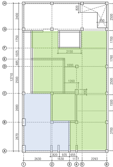
Lantai Lt I
