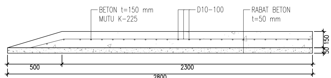
POTONGAN B SKALA 1 : 20
