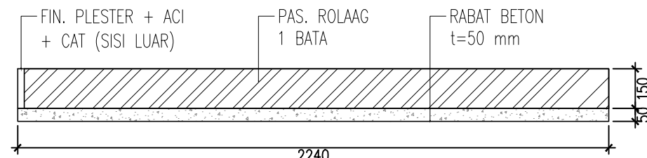
POTONGAN A SKALA 1 : 20
